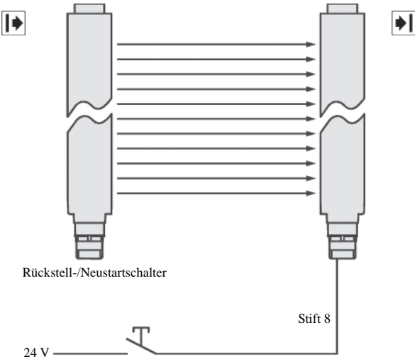
Abbildung 15: Rückstell-/Neustartschalter verbinden
