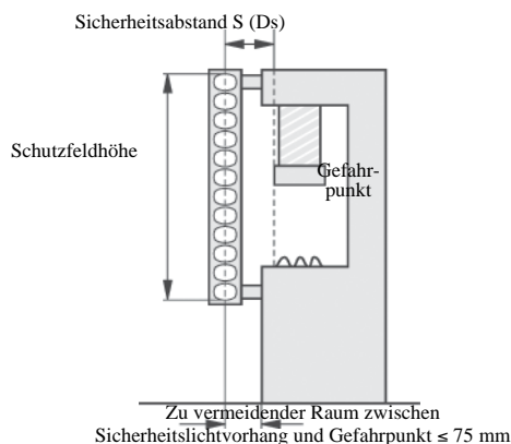
Abbildung 4: Sicherheitsabstand vom Gefahrpunkt
