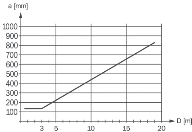
Abbildung 6: Graph, Mindestabstand von reflektierenden Oberflächen
