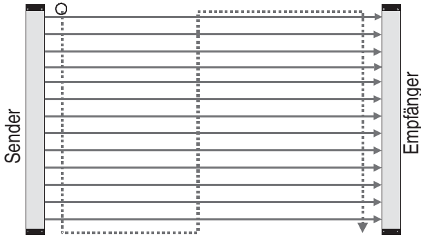
Abbildung 16: Test des Schutzfelds mit dem Teststab
