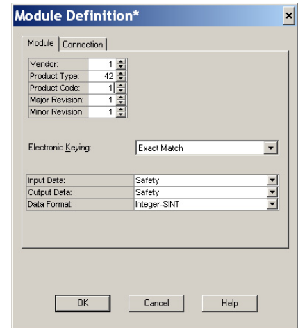
1734-IE4S Module
